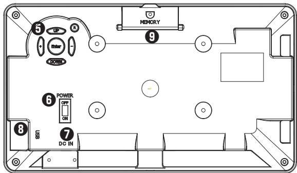
⑤ 操作ボタン(十字キー) ⑥ 電源スイッチ (ON / OFF) ⑦ DC IN電源プラグ ⑧ USB2.0接続端子 ⑨ SDメモリーカードスロット
