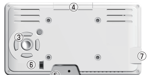
③ 操作ボタン(十字キー) ⑤ DC IN (電源コネクタ) ④ SD メモリーカードスロット ⑥ POWER (電源スイッチ) ⑦ USB2.0 接続端子
