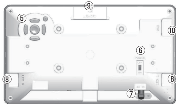
⑤ 操作ボタン (十字キー) ⑥ POWER (電源スイッチ) ⑦ DC IN (電源コネクタ) ⑧ LED OUT 端子 (L/R) ⑨ SDメモリーカードスロット ⑩ USB2.0 接続端子
