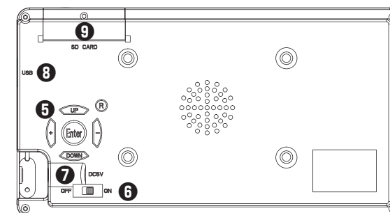
⑤ 操作ボタン(十字キー) ⑧ USB2.0接続端子 ⑥ 電源スイッチ (ON / OFF) ⑨ SDメモリーカードスロット ⑦ DC IN電源プラグ
