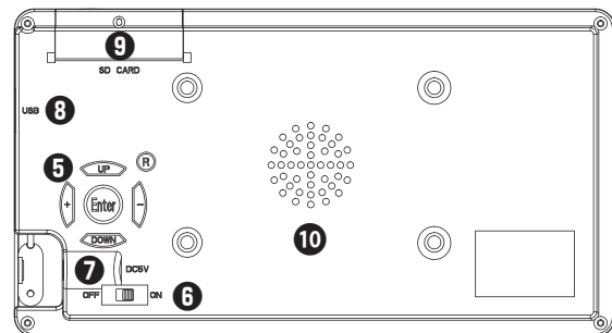
⑤ 操作ボタン(十字キー) ⑧ USB2.0接続端子 ⑥ 電源スイッチ(ON / OFF) ⑨ SDメモリーカードスロット ⑦ DC IN電源プラグ ⑩ スピーカー
